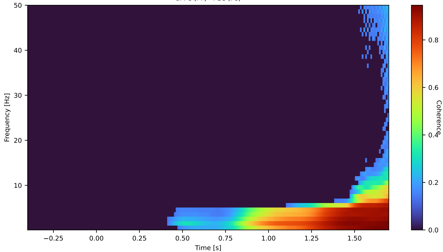
dPFC (F7) - PEC (P8)
